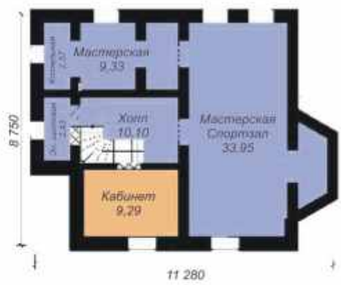
План цокольного этажа
