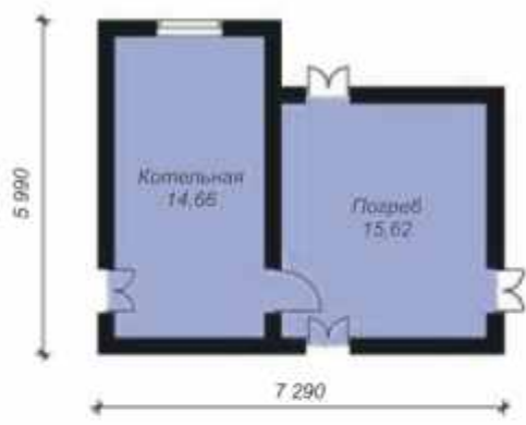
План цокольного этажа
